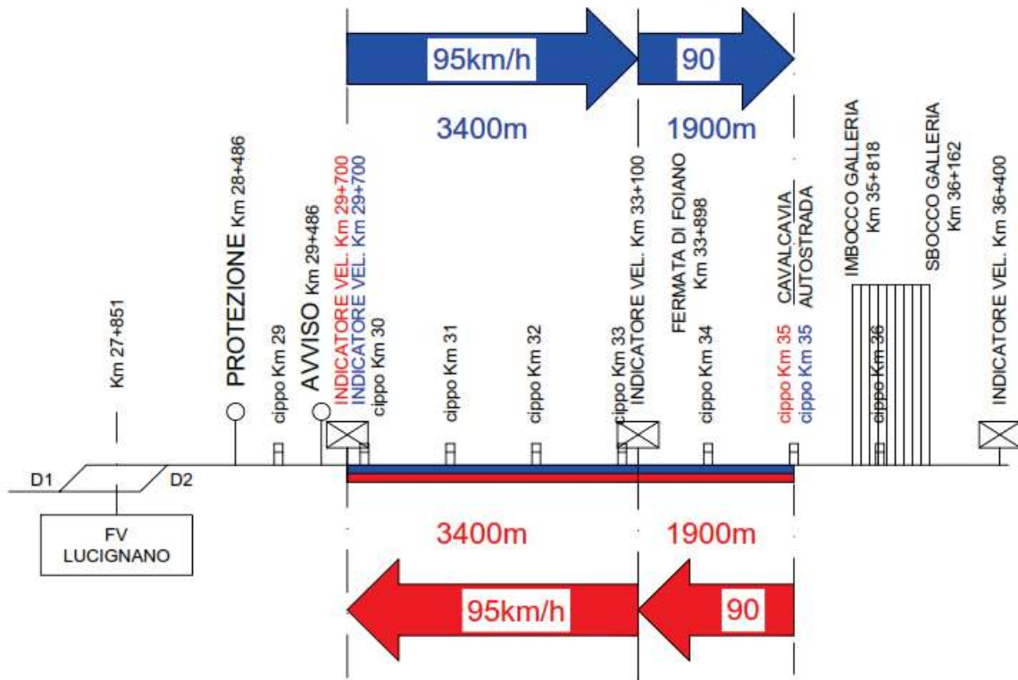
Individuazione delle tratte di prova tra le stazioni di Lucignano LFI e di Sinalunga RFI.
